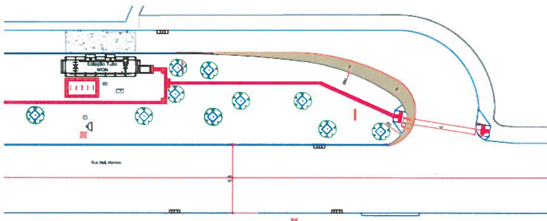
Figura 3: Estação Museu Oscar Niemeyer – Estação existente correção geométrica a executar. Fonte: URBS, 2017
