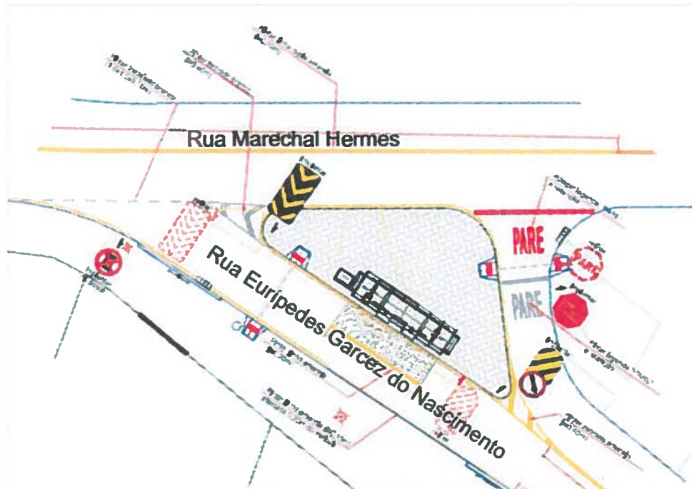
Figura 2: Estação Museu Oscar Niemeyer – Estação tubo a implantar Fonte: URBS, 2017
