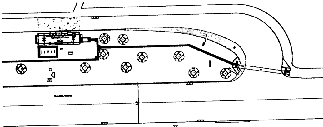
Figura 3: Estação Museu Oscar Niemeyer – Estação existente correção geométrica a executar. Fonte: URBS, 2017
